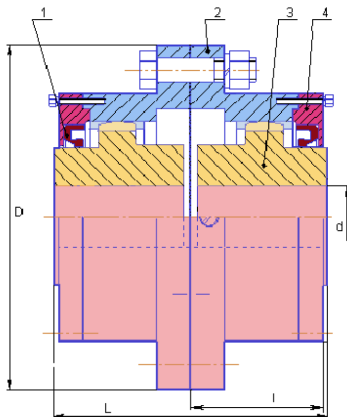
Муфта зубчатая МЗ: составные части и основные размеры
